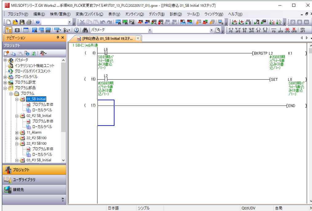
図 7-13 変更前「01_SB Initial」ラダープログラム
