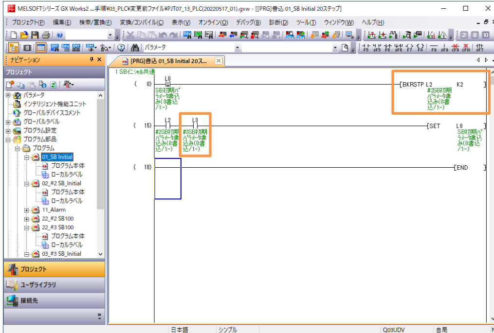
図 7-14 変更後「01_SB Initial」ラダープログラム
