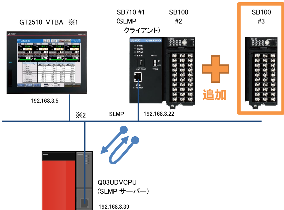
図 3-1 機器構成図
