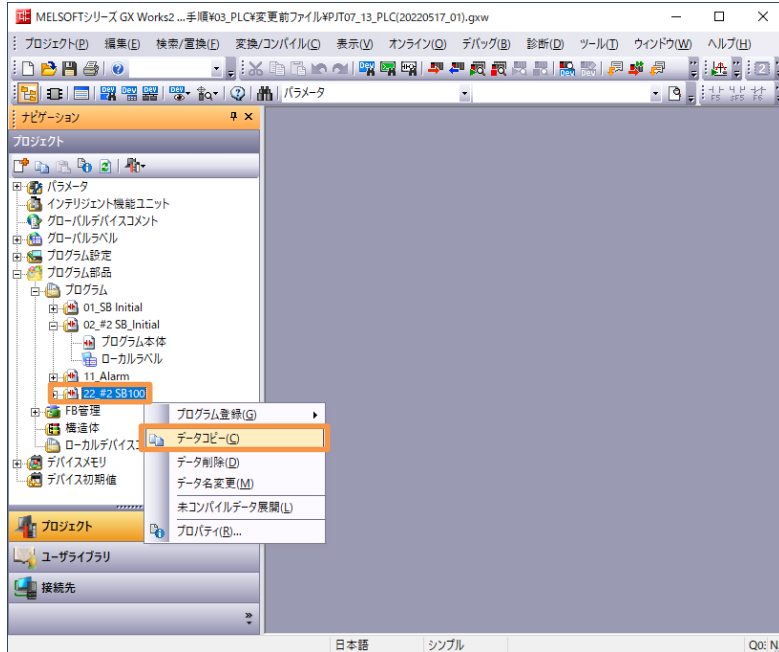
図 7-1「22_#2 SB100」プログラムコピー
