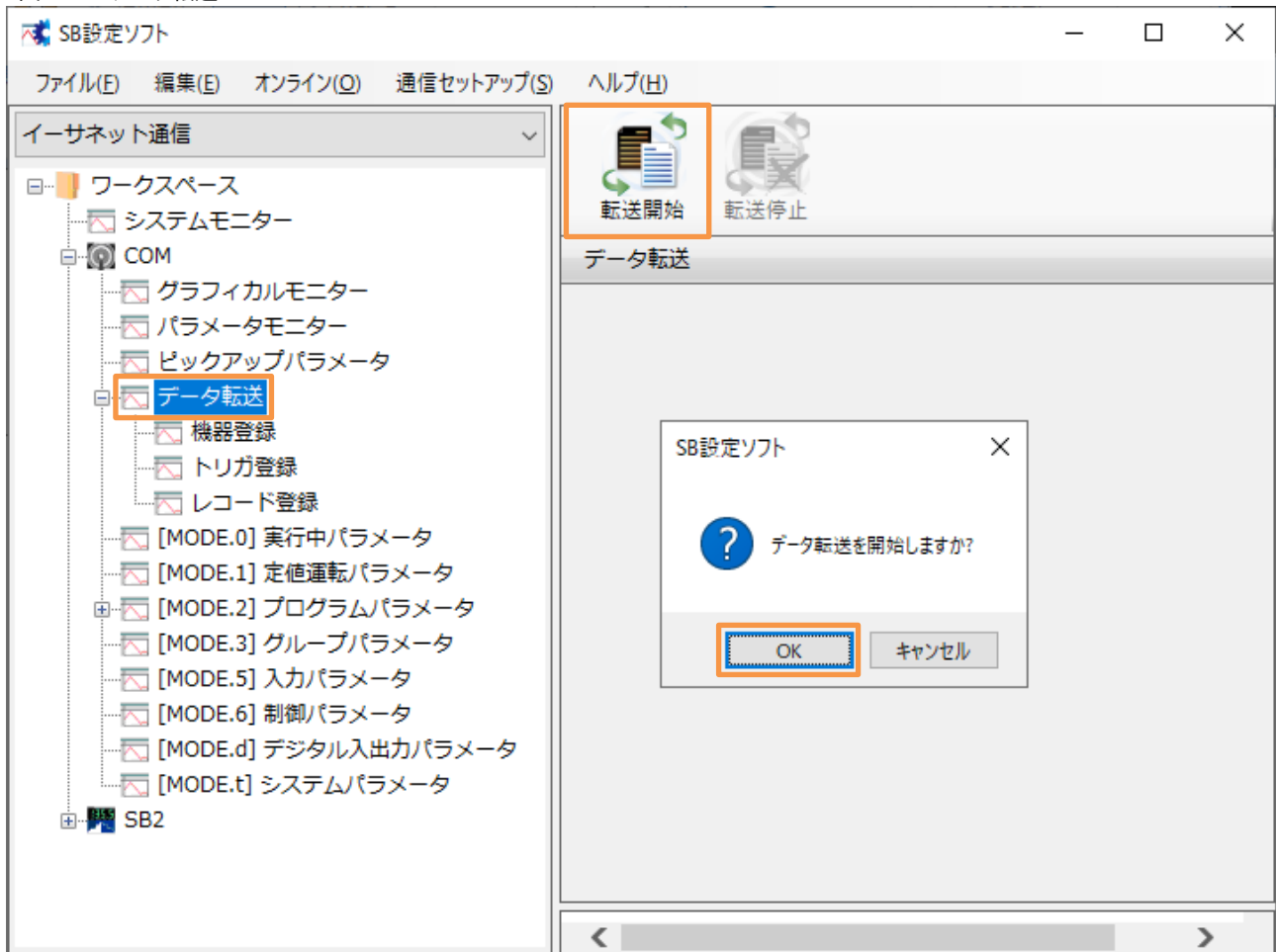
図 6-15 データ転送
